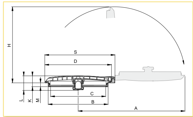
Versione senza bloccaggio di chiusura Version without lockup blocking Versión sin bloqueo de cierre
