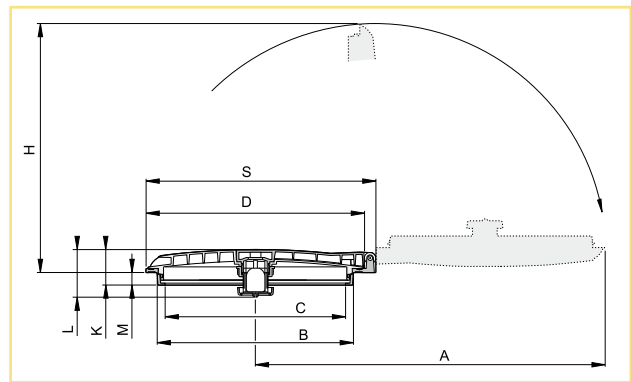
Versione con bloccaggio di chiusura Version with lockup blocking Versión con bloqueo de cierre
